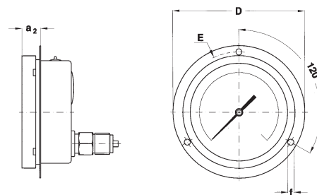
Е - ПЕРЕДНИЙ ФЛАНЕЦ, для осевого присоединения
